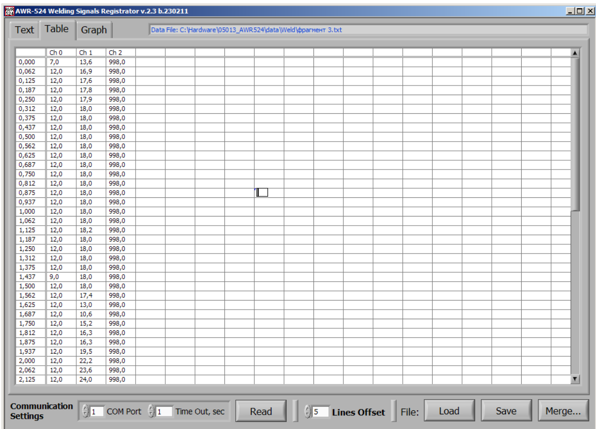
Рис. 4. Окно программы – Вкладка «Данные в форме таблицы»
