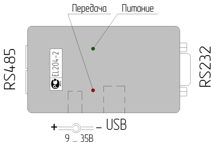
Рисунок 2 – Расположение разъёмов и индикации
