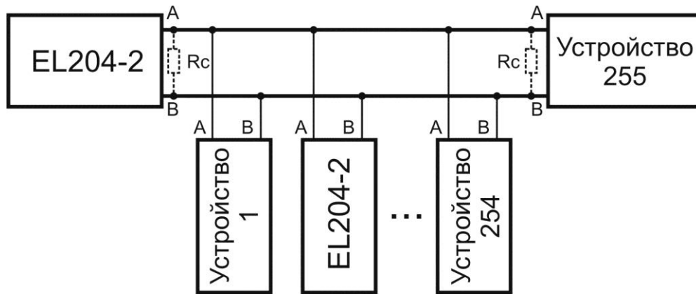
Рисунок 9 – Схема подключения преобразователя к сети RS485
